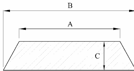
شکل ۸-۴- ابعاد ریشه
