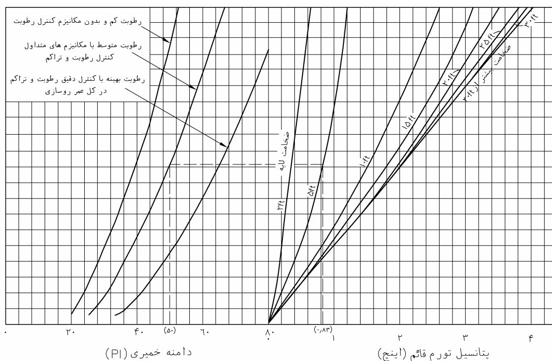
شکل پ-۱-۲- نمودار تعیین بالآمدگی قائم خاک بستر
