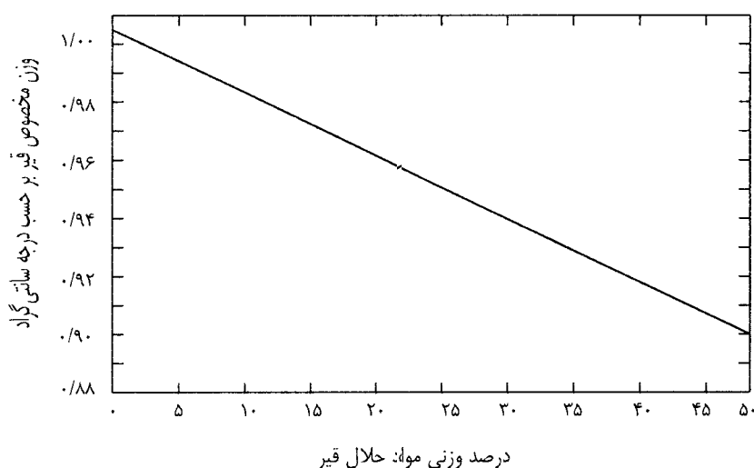
شکل (۷-۴): تغییرات وزن مخصوص یک نمونه قیر در ۵ درجه سانتیگراد بر حسب میزان مواد حلال موجود در آن [۱۱]
