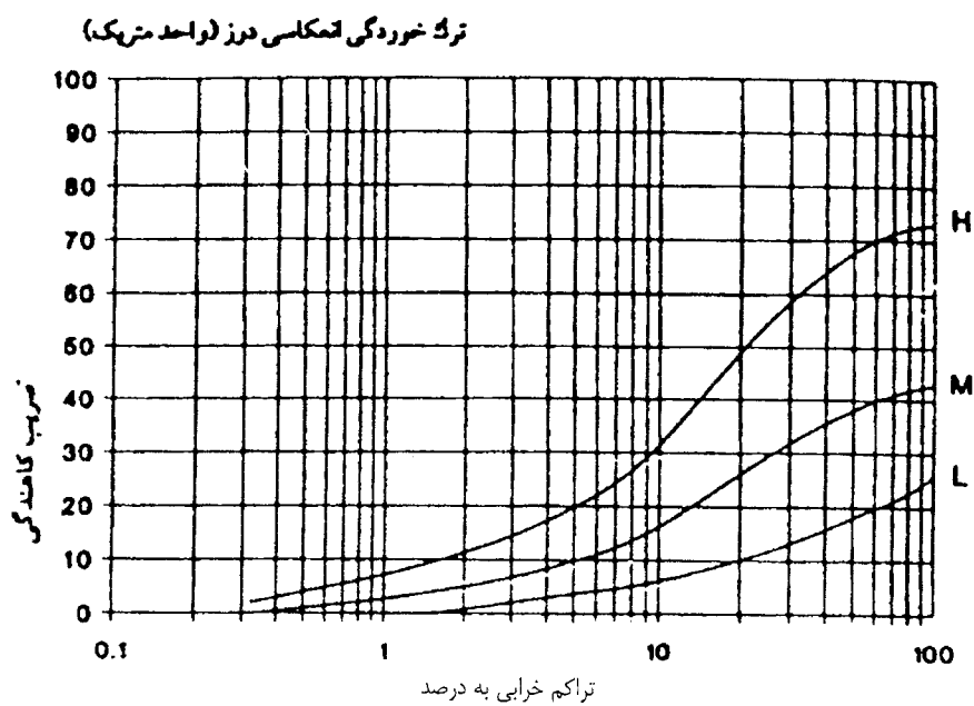
شکل (۱-۶-پ): منحنی ضریب کاهندگی برای خرابی از نوع ترک خوردگی انعکاسی
