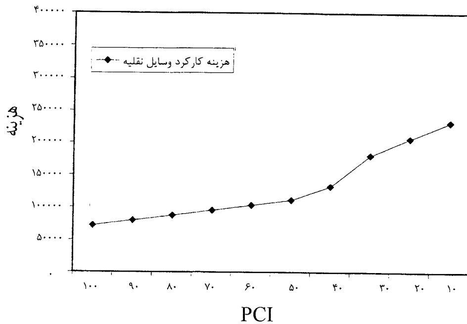
شکل (۷-۹): نمودار هزینه کارکرد وسایل نقلیه به تفکیک در سرعت ۶۰ کیلومتر بر ساعت
