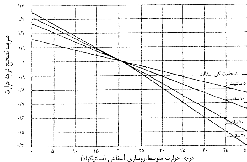
شکل (۸-۴): ضریب تصحیح درجه حرارت بر حسب درجه حرارت متوسط روسازی آسفالتی [۱۱]
