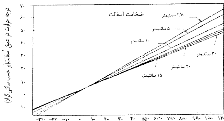
شکل (۸-۳): تعیین درجه حرارت متوسط لایه آسفالت روسازی در آزمایش افت‌وخیز [۱۱]
