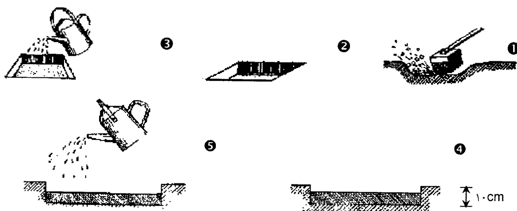
شکل (۵-۲) - مراحل اجرایی لکه‌گیری
