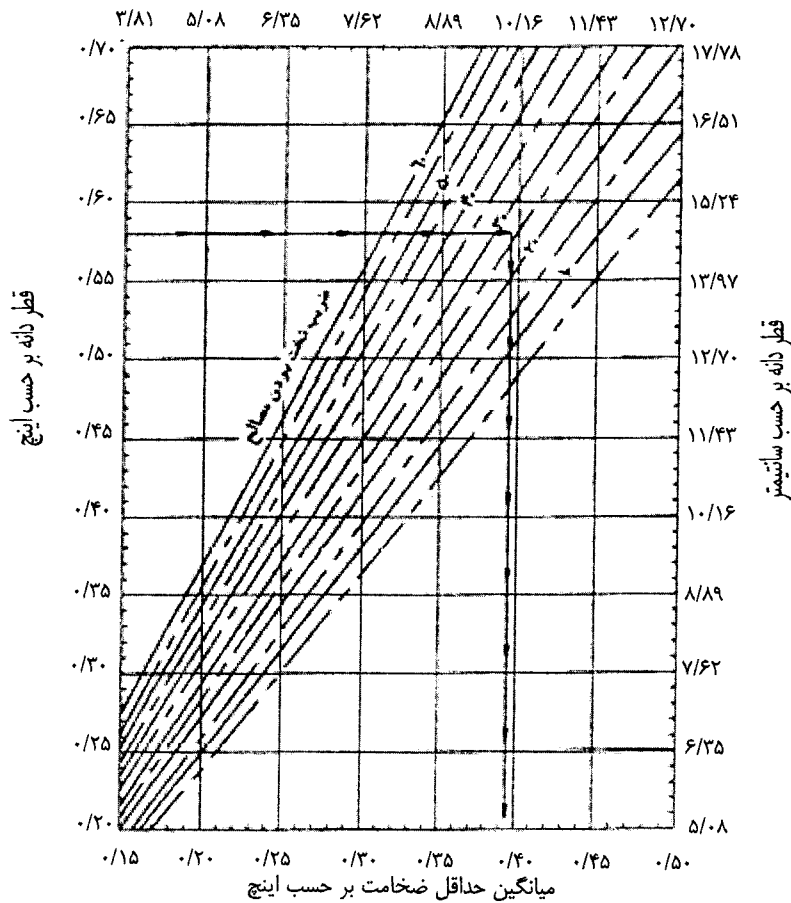
شکل (۲-۷): تعیین میانگین کمترین بعد سنگدانه‌ها [۱۱]
