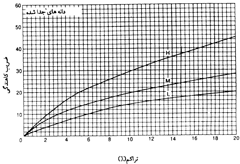
شکل (۲-۶-پ): منحنی ضریب کاهندگی برای خرابی از نوع شیارشدگی
