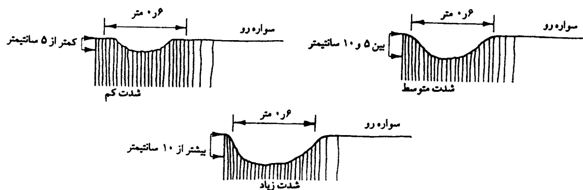
شکل (۵-۳): چاله
