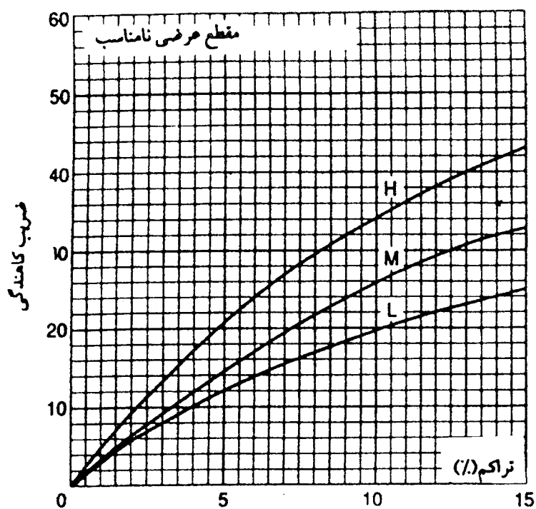
شکل (۲-۱-پ): منحنی ضریب کاهندگی برای خرابی از نوع مقطع عرضی نامناسب
