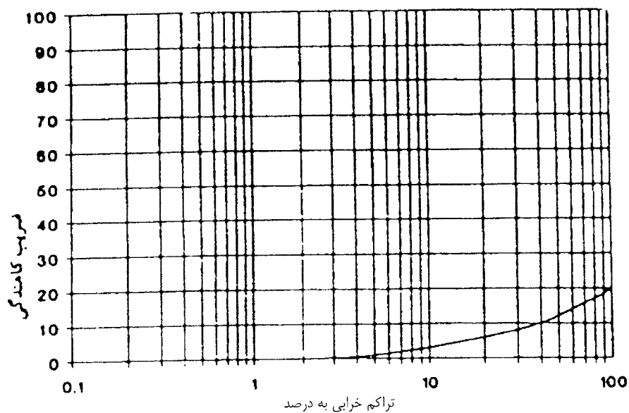
شکل (۱-۱۰-پ): منحنی ضریب کاهندگی برای خرابی از نوع صیقلی شدن دانه ها
