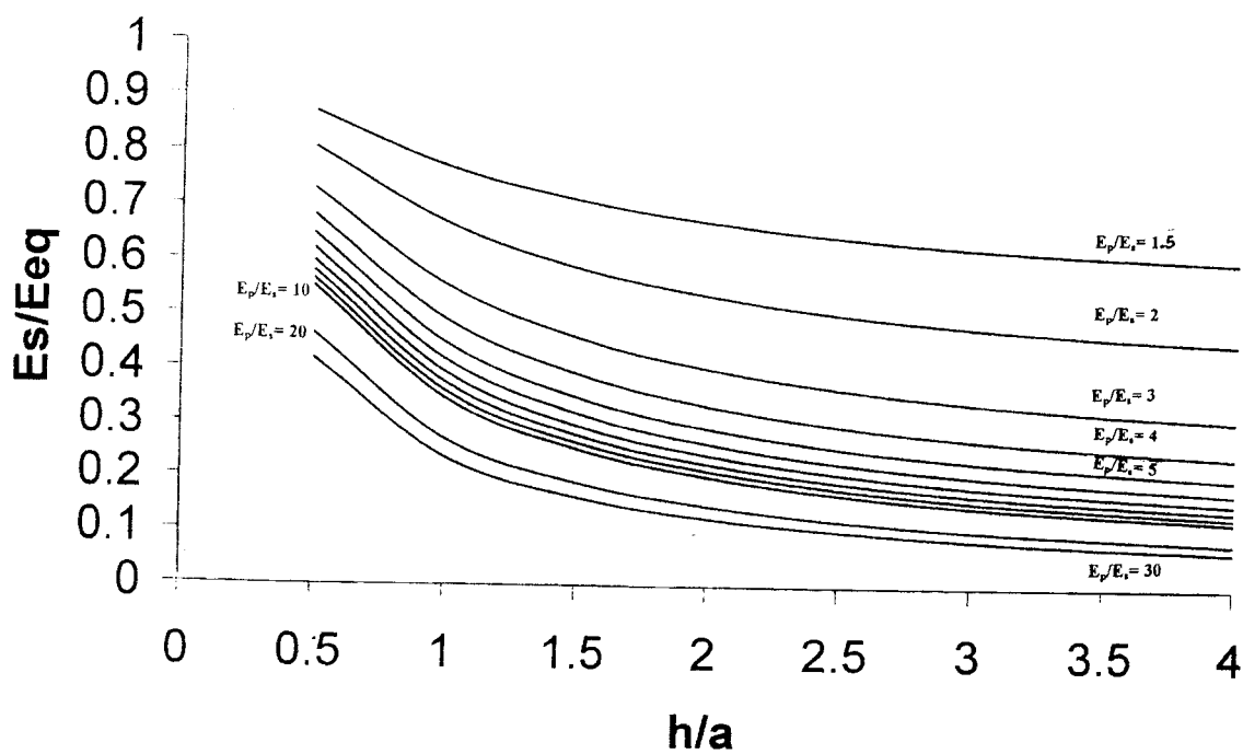
شکل (۴-۳) پ) نمودار تعیین مدول روسازی با \mu_P = 0.5 , \mu_S = 0.35
