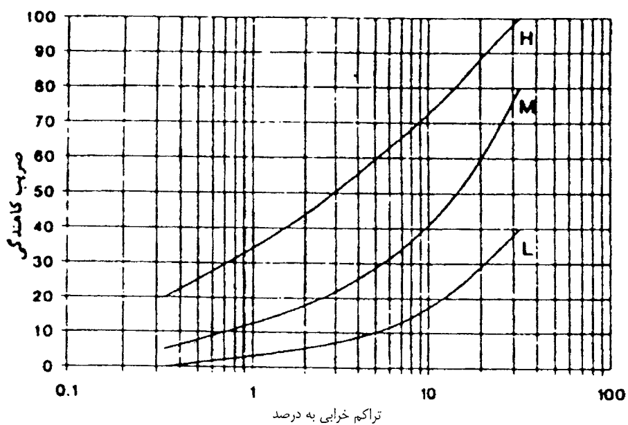
شکل (۱-۲-پ): منحنی ضریب کاهندگی برای خرابی از نوع برآمدگی و فرورفتگی
