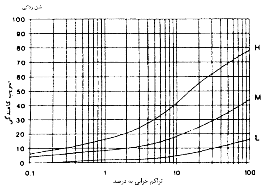
شکل (۱-۱۹-پ): منحنی ضریب کاهندگی برای خرابی از نوع شن زدگی
