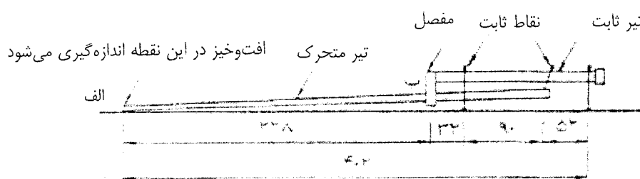
شکل (۲-۸): تصویر کلی تیر بشکل من (اندازه‌ها بر حسب سانتیمتر) [۱۱]
