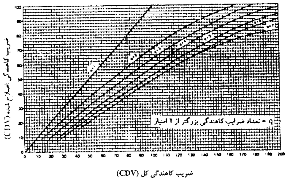
شکل (۱-۲۰-پ): منحنی ضریب کاهندگی کل برای راههای رویه‌دار
