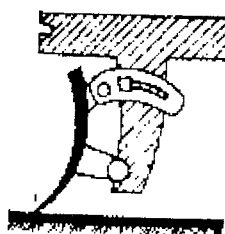
شکل (۵-۶) نحوه بستن تیغه‌گریدر
