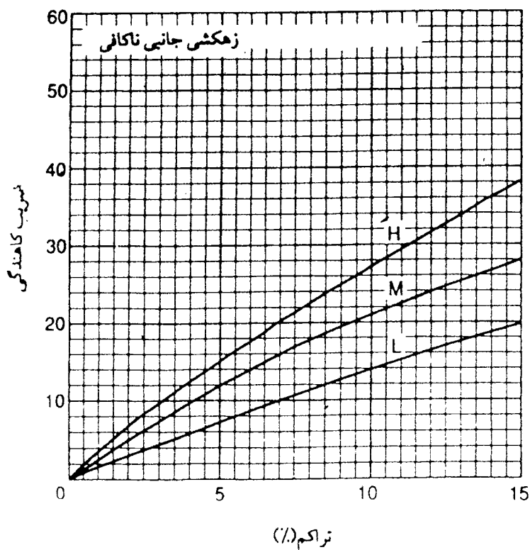
شکل (۲-۲-پ): منحنی ضریب کاهندگی برای خرابی از نوع زهدکشی جانی ناکافی
