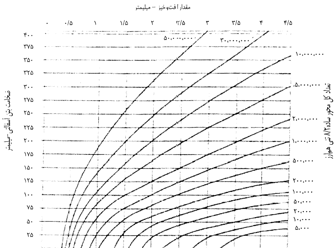
شکل (۷-۸) تعیین ضخامت روکش آسفالت بر حسب آزمایش افت‌وخیز
