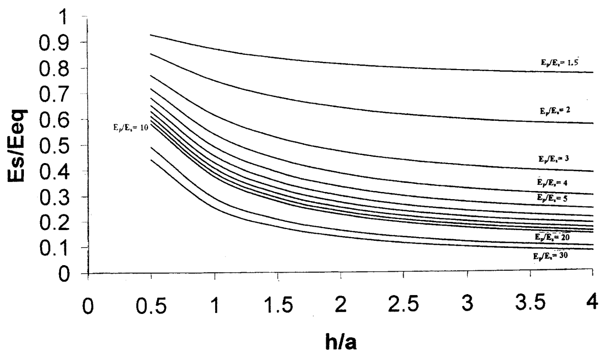
شکل (۴-۸ پ): نمودار تعیین مدول معادل روسای با \mu_p = 0.25 , \mu_s = 0.45
