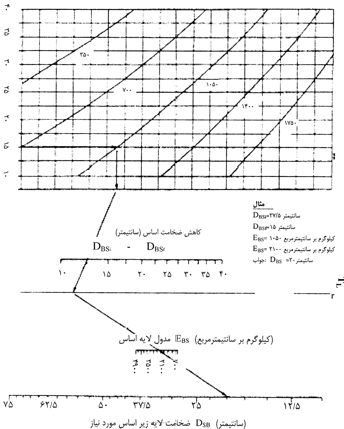
شکل (۵-۱۲): نمودار تبدیل بخشی از ضخامت لایه اساس به ضخامت لایه زیر اساس معادل [۲۳]
