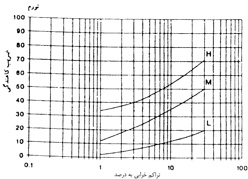
شکل (۱-۱۶-پ): منحنی ضریب کاهندگی برای خرابی از نوع تورم
