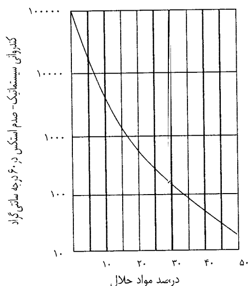
شکل (۷-۶): نمودار کندروانی نمونه‌ای از یک قیر محلول حاوی درصد‌های مختلف مواد حلال [۱۱]
