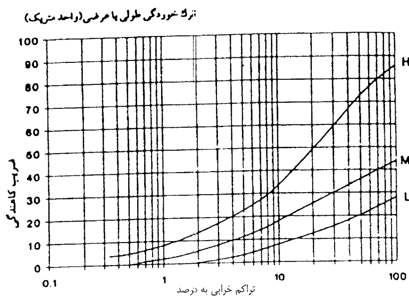
شکل (۸-۱-پ): منحنی ضریب کاهندگی برای خرابی از نوع ترک خوردگی طولی یا عرضی
