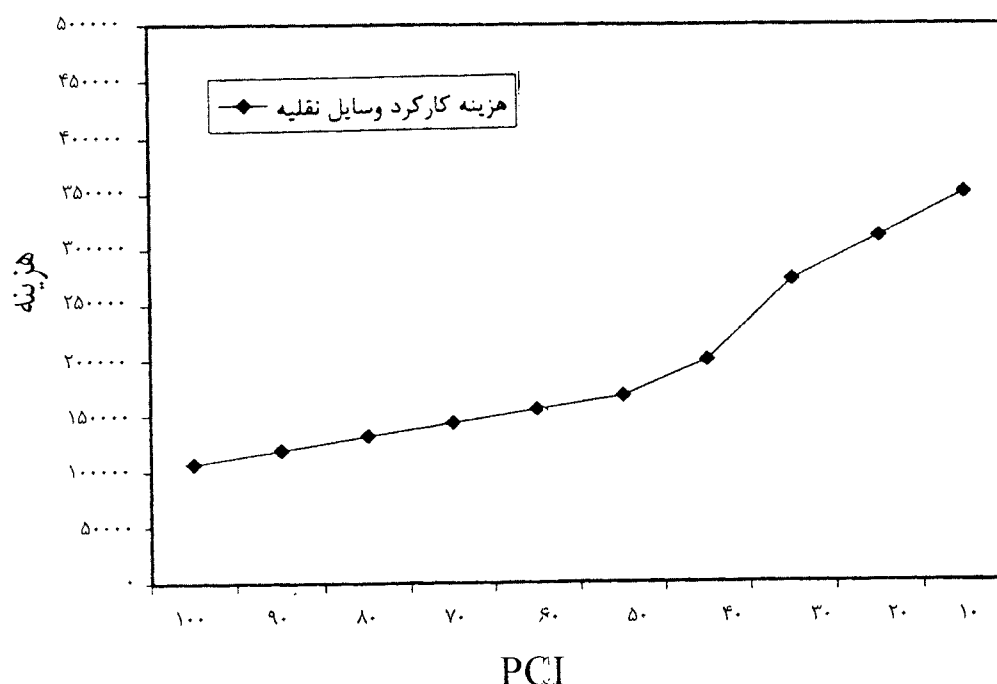
شکل (۹-۹): نمودار هزینه کارکرد وسایل نقلیه به تفکیک در سرعت ۱۲۰ کیلومتر بر ساعت
