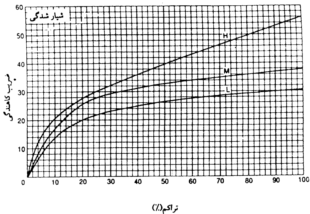
شکل (۲-۶-پ): منحنی ضریب کاهندگی برای خرابی از نوع شیارشدگی
