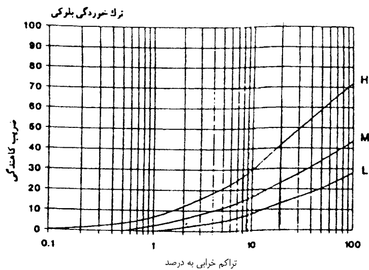
شکل (۱-۱-پ): منحنی ضریب کاهندگی برای خرابی از نوع ترک خوردگی
