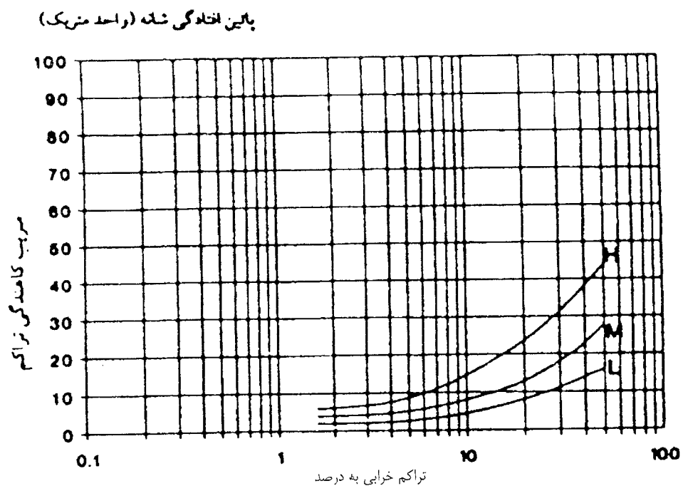
شکل (۷-۱-پ): منحنی ضریب کاهندگی برای خرابی از نوع پایین افتادگی شانه
