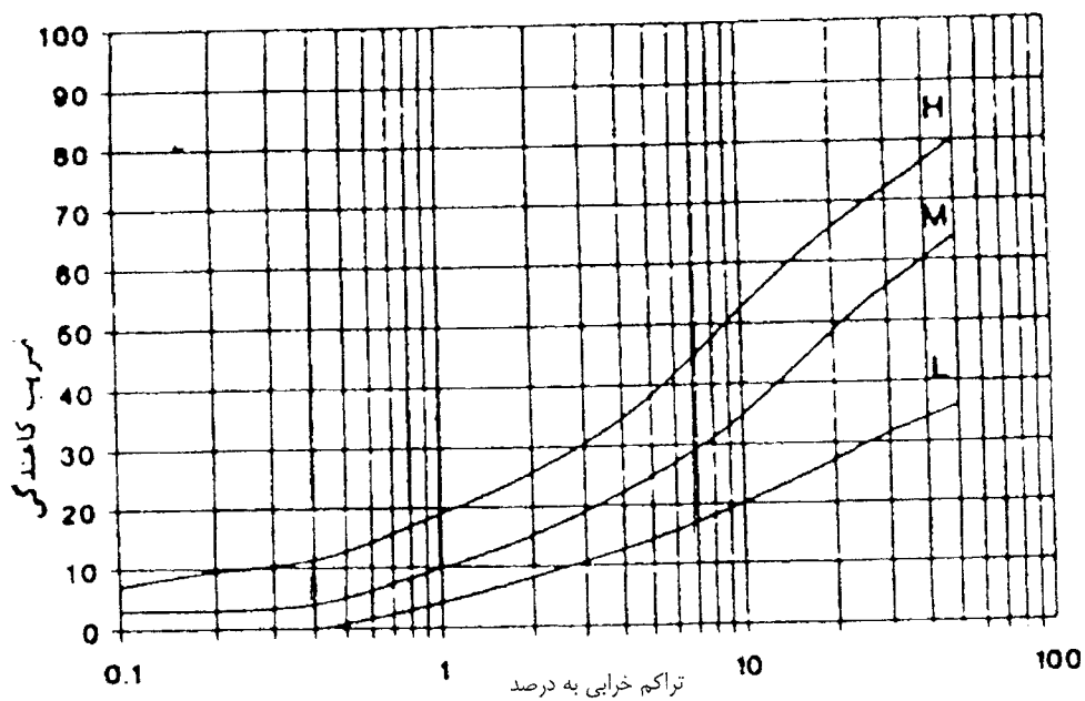
شکل (۱-۱۴-پ): منحنی ضریب کاهندگی برای خرابی از نوع کنارزدگی
