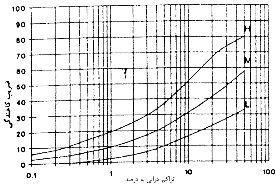
شکل (۱-۹-پ): منحنی ضریب کاهندگی برای خرابی از نوع وصله و کنده کاری
