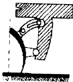
ب) حالت تیغه‌گریدر در موقع پخش و تسطیح
