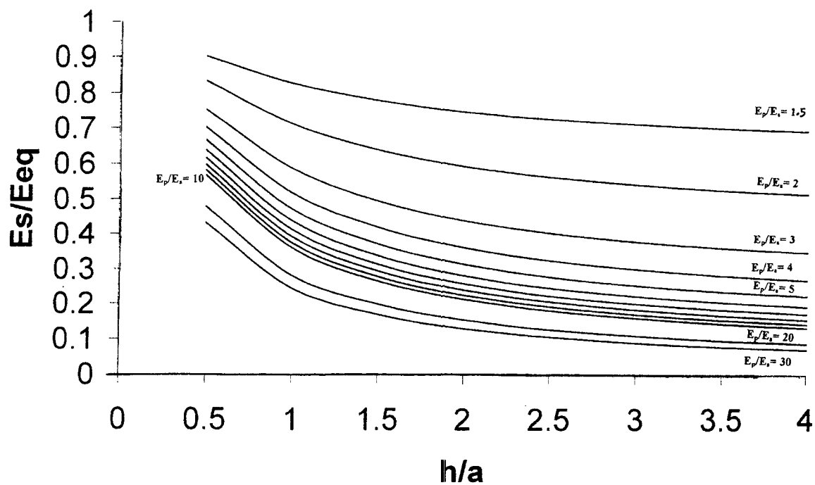
شکل (۴-۹) نمودار تعیین مدول معادل، روسازی با \mu_p = 0.25 , \mu_s = 0.35
