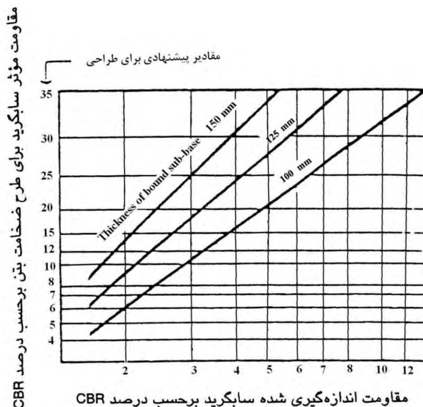
شکل ۳۹ اثرات زیر اساس غیر چسبنده بر روی مقاومت طراحی ساگرید (CBR)
