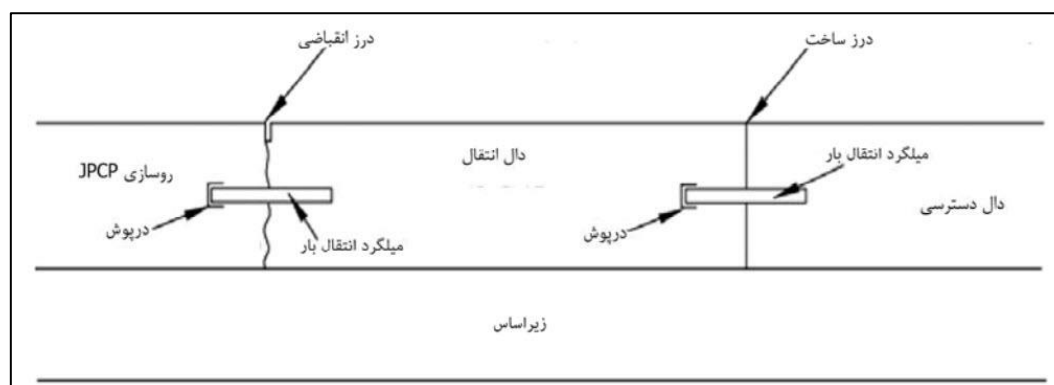
شکل ۲۲ جزئیات اجرای ناحیه انتقال روسازی های بتنی و دال دسترسی پل با استفاده از دال با ضخامت ثابت
