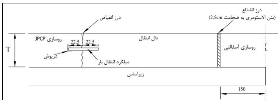
شکل ۲۱ جزئیات اجرایی ناحیه انتقال روسازی های بتنی و آسفالتی با استفاده از درز انقطاع با پرکننده بتن
